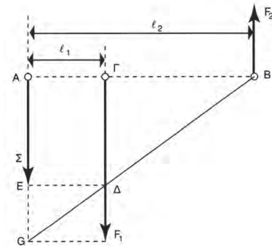
Σχήμα 3.8α Η γραφική μέθοδος
