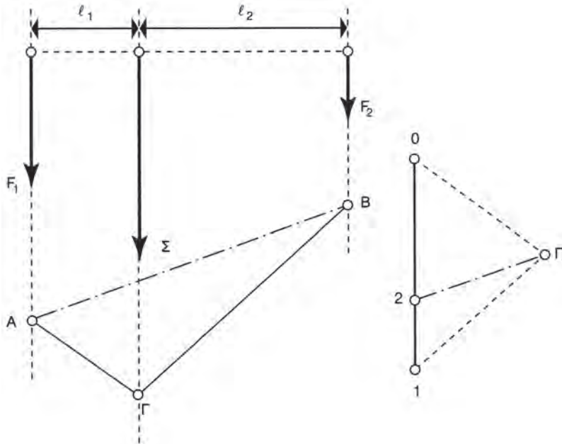
Σχήμα 3.7β Δεύτερη γραφική μέθοδος
